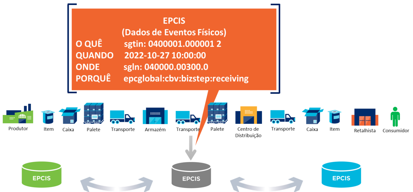
Figura 4. Dados de Eventos Físicos através de GS1® EPCIS
